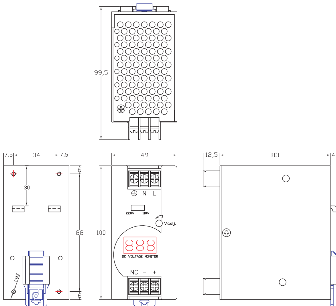
機 構 圖
