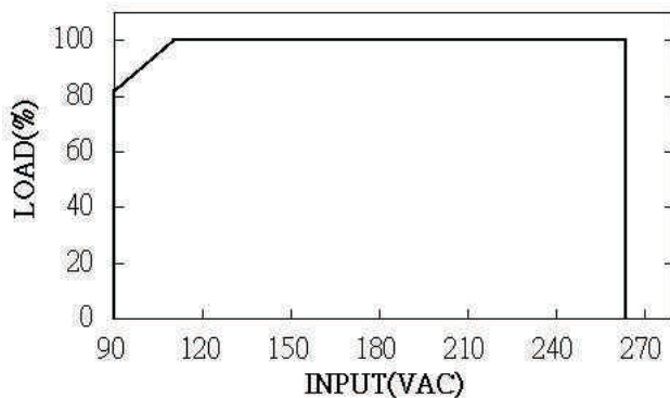
降額曲線
